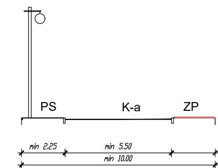
UK2 - presjek 2-2
