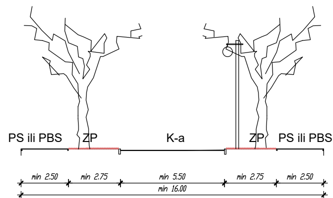
UK1 - presjek 1-1
