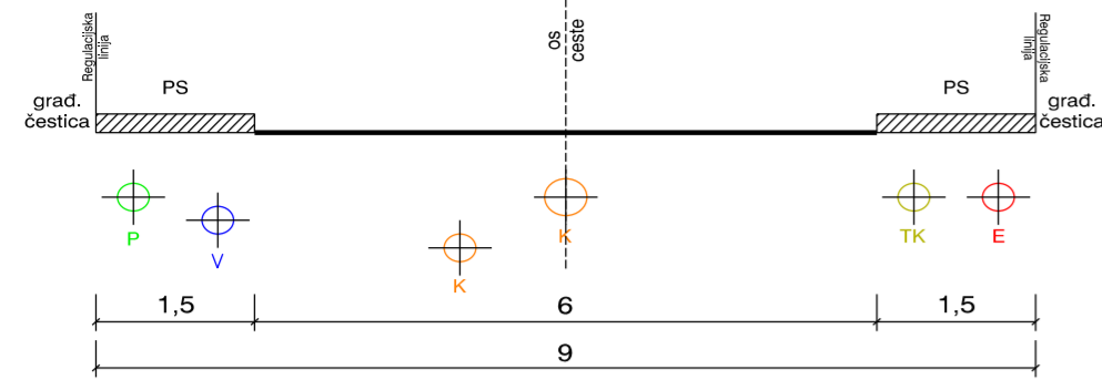
PRESJEK 3-3
