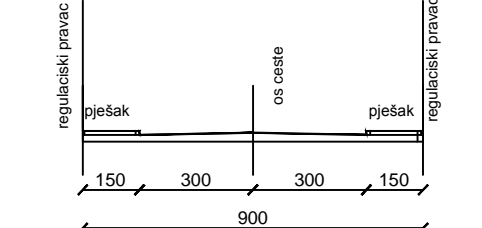
KARAKTERISTIČAN POPREČNI PRESJEK A' - A' M 1:200
