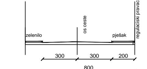
KARAKTERISTIČAN POPREČNI PRESJEK B - B M 1:200
