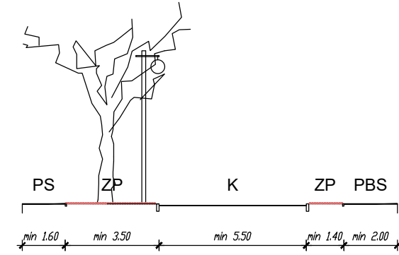
UK1 - presjek 1-1
