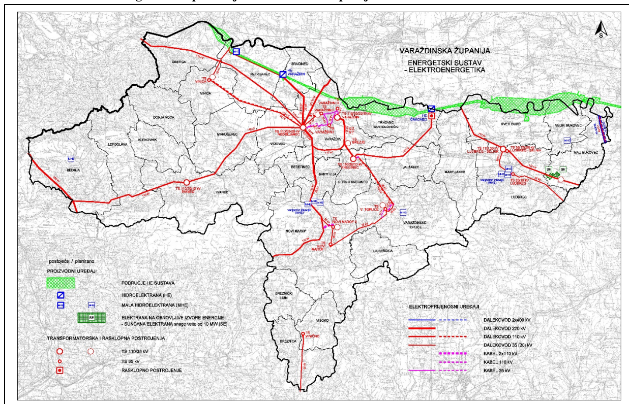
Slika 2. - Elektroenergetika na području Varaždinske županije
