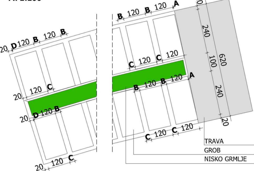
DETALJ PRIKAZA RASPOREDA UKOPNIH MJESTA U KARAKTERISTIČNOM REDU GROBNOG POLJA M. 1:100
