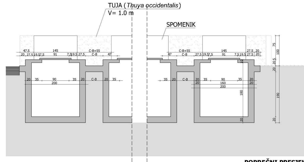
POPREČNI PRESJEK
