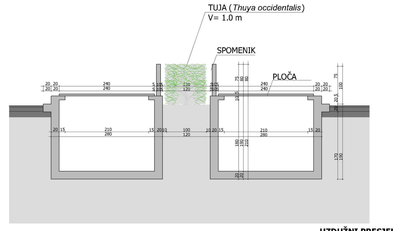
UZDUŽNI PRESJEK
